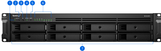
전면(RS1221RP+)
