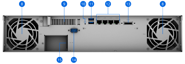
후면(RS1221RP+)
