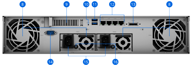
후면(RS1221RP+)
