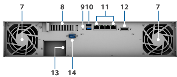
Zadní část
