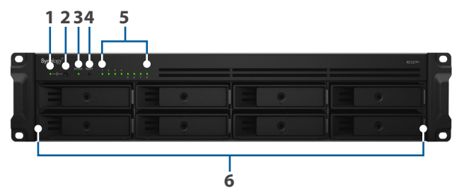
Přední část
