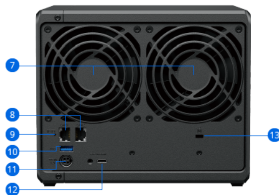
Achterkant
