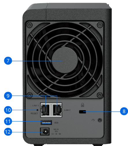
DS224+ (hátnézet)
